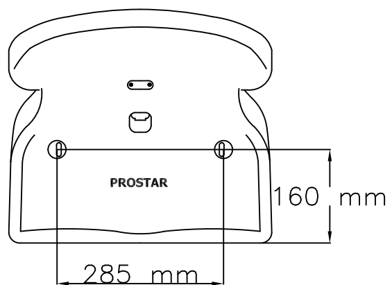
POGLED ODOZGO
