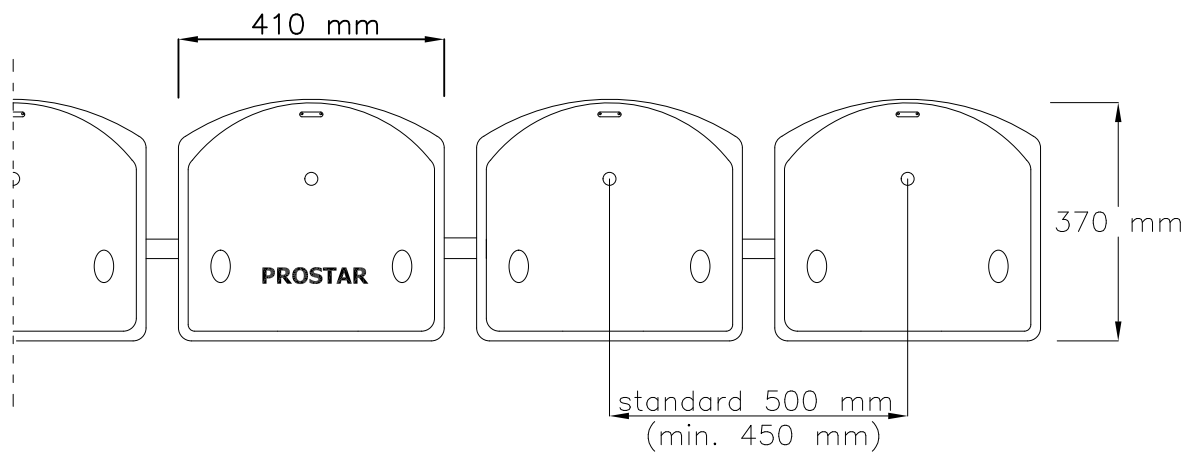
POGLED ODOZGO
