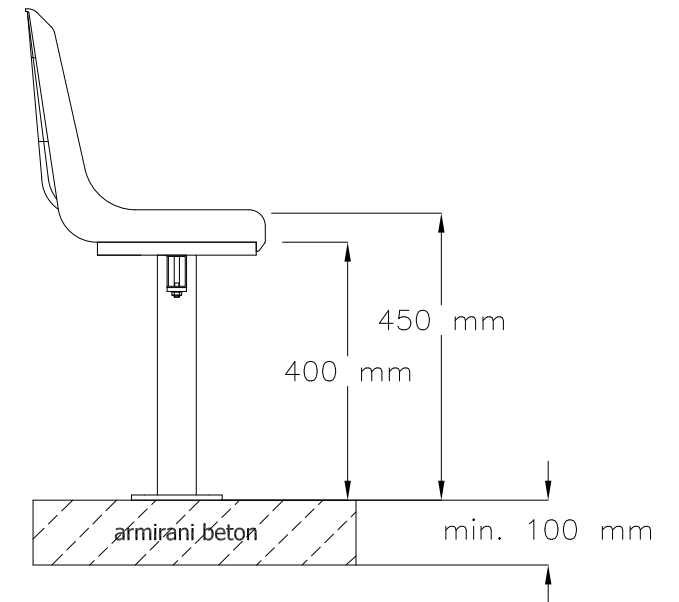
BOČNI POGLED
