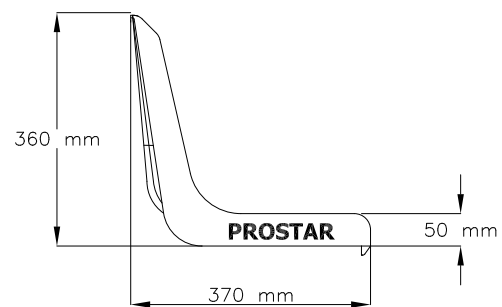
BOČNI POGLED
