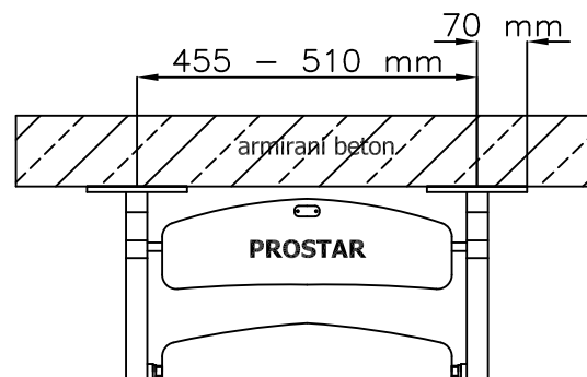
POGLED ODOZGO
