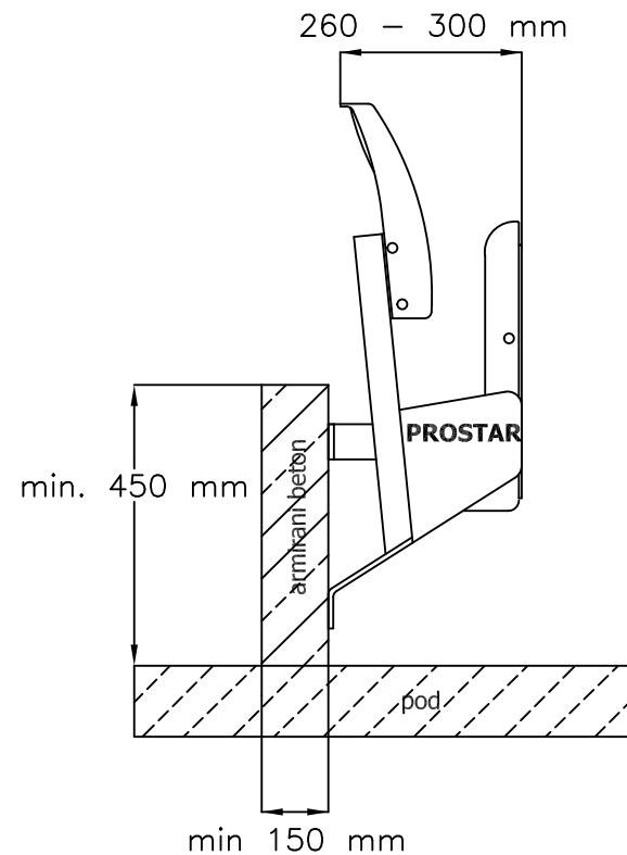
BOČNI POGLED
