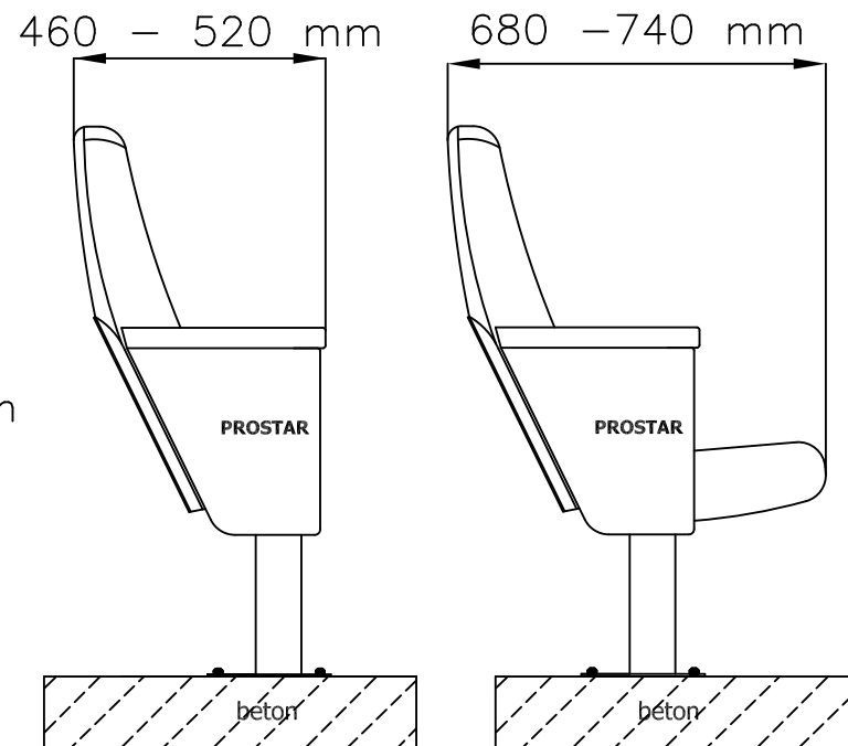
BOČNI POGLED
